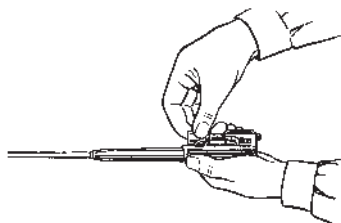
Рис. 20. Отделение затвора от затворной рамы
