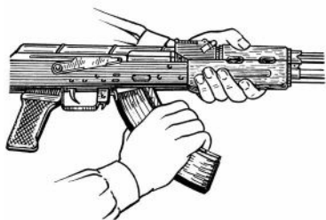
Рис. 15. Отделение магазина
