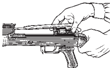
Рис. 19. Отделение затворной рамы с затвором
