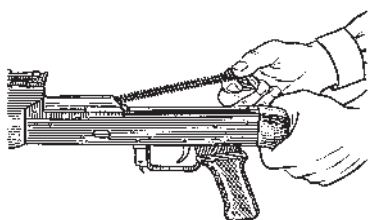
Рис. 18. Отделение возвратного механизма
