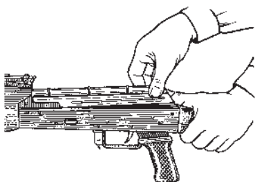
Рис. 17. Отделение крышки ствольной коробки
