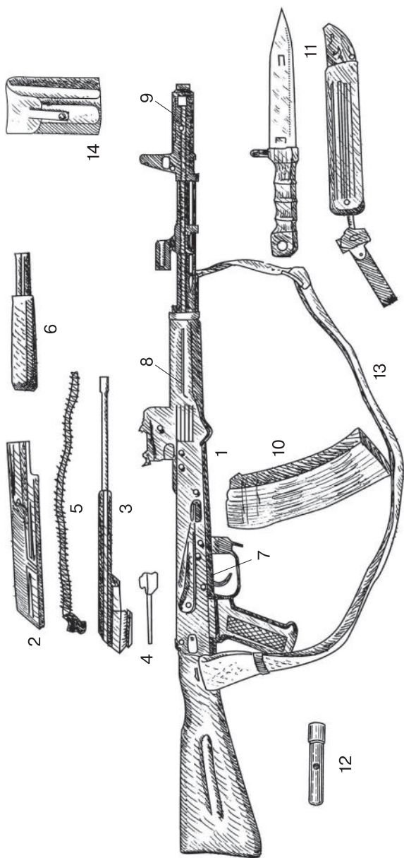
Рис. 14. Основные части и механизмы автомата:
