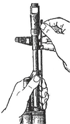
Отделение шомпола
