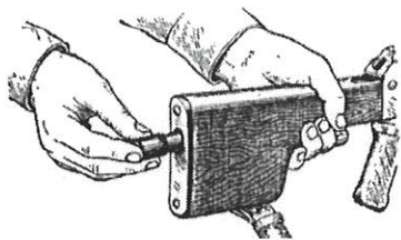
Вкладывание пенала принадлежности в гнездо приклада
