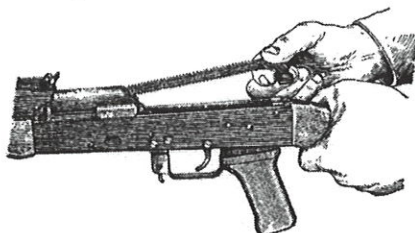
Отделение возвратного механизма
